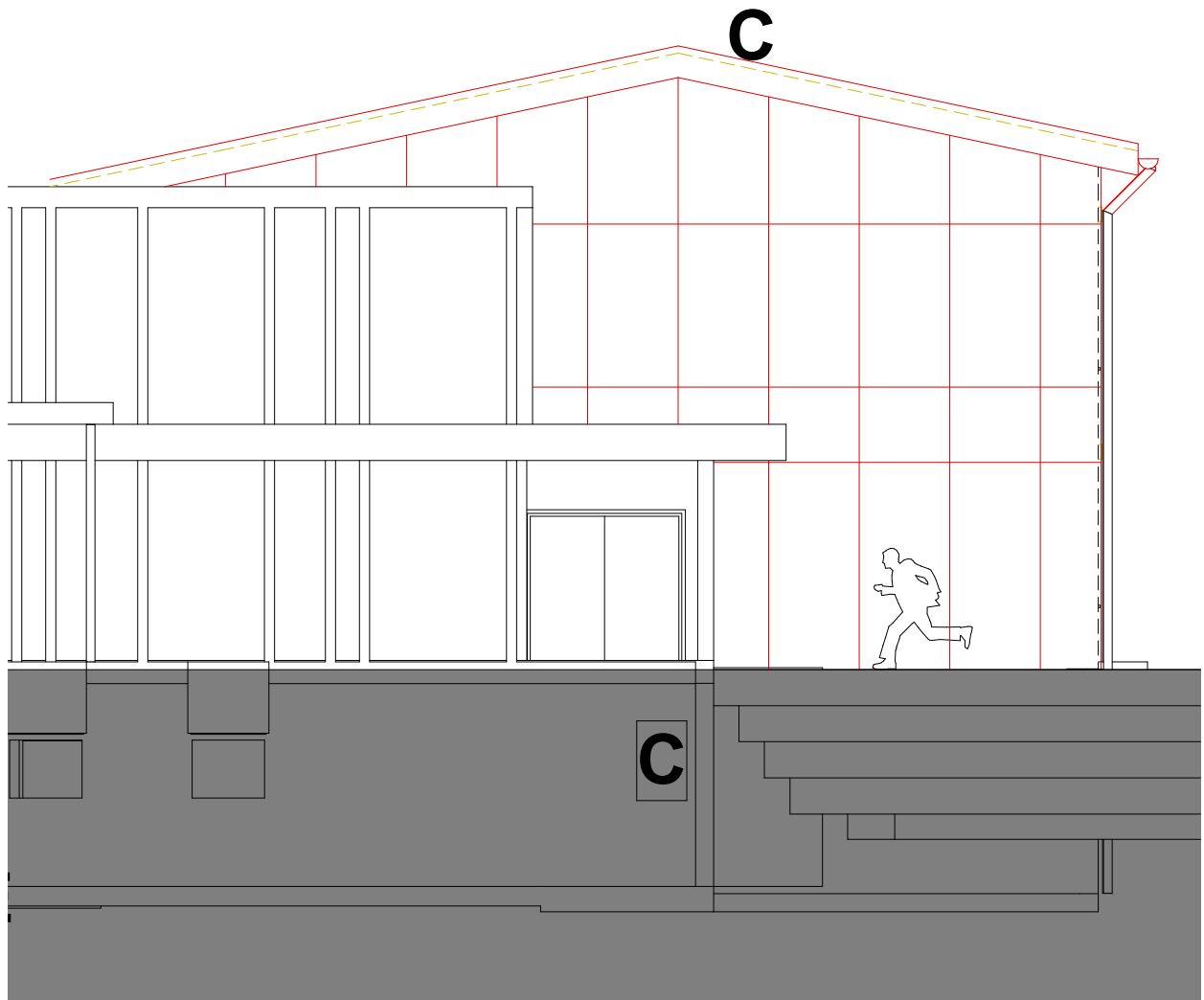
Fassade Südwest M 1:100
